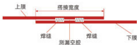
LST-GM1 焊接示意图
